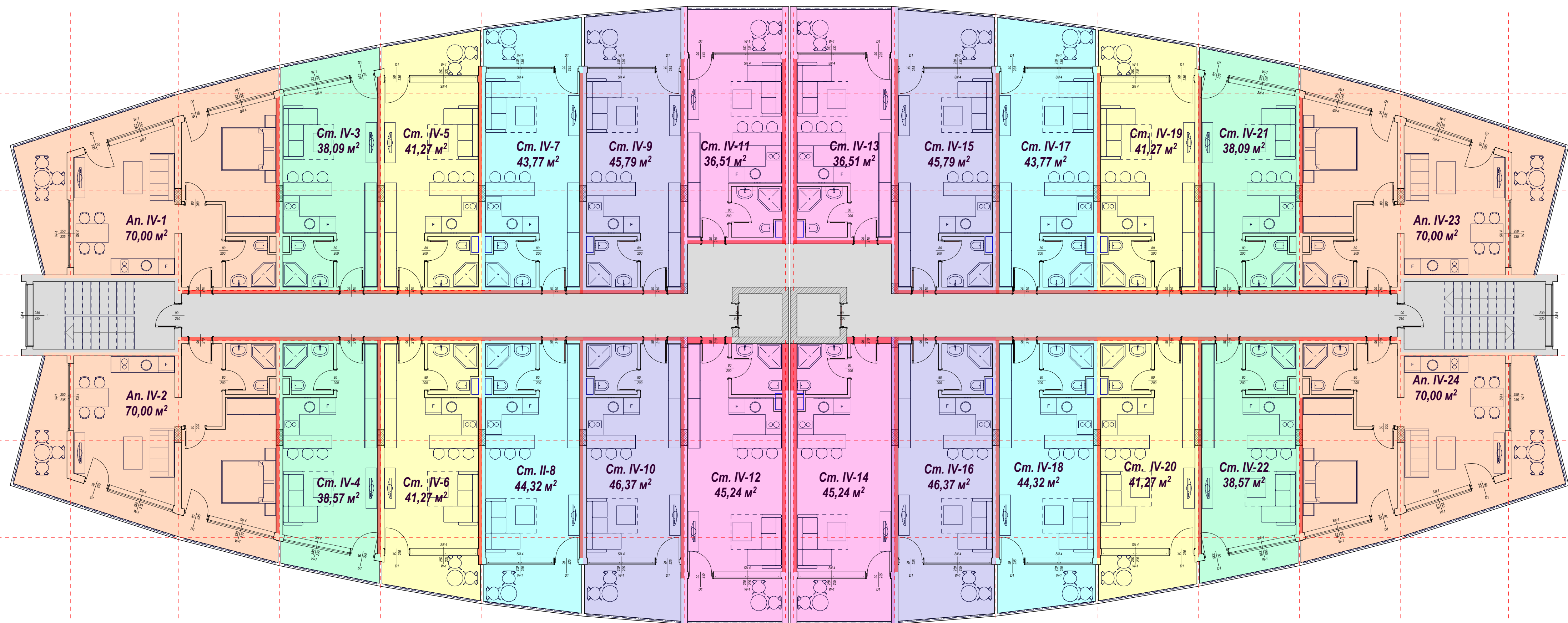
РАЗПРЕДЕЛЕНИЕ КОТА +8,37
