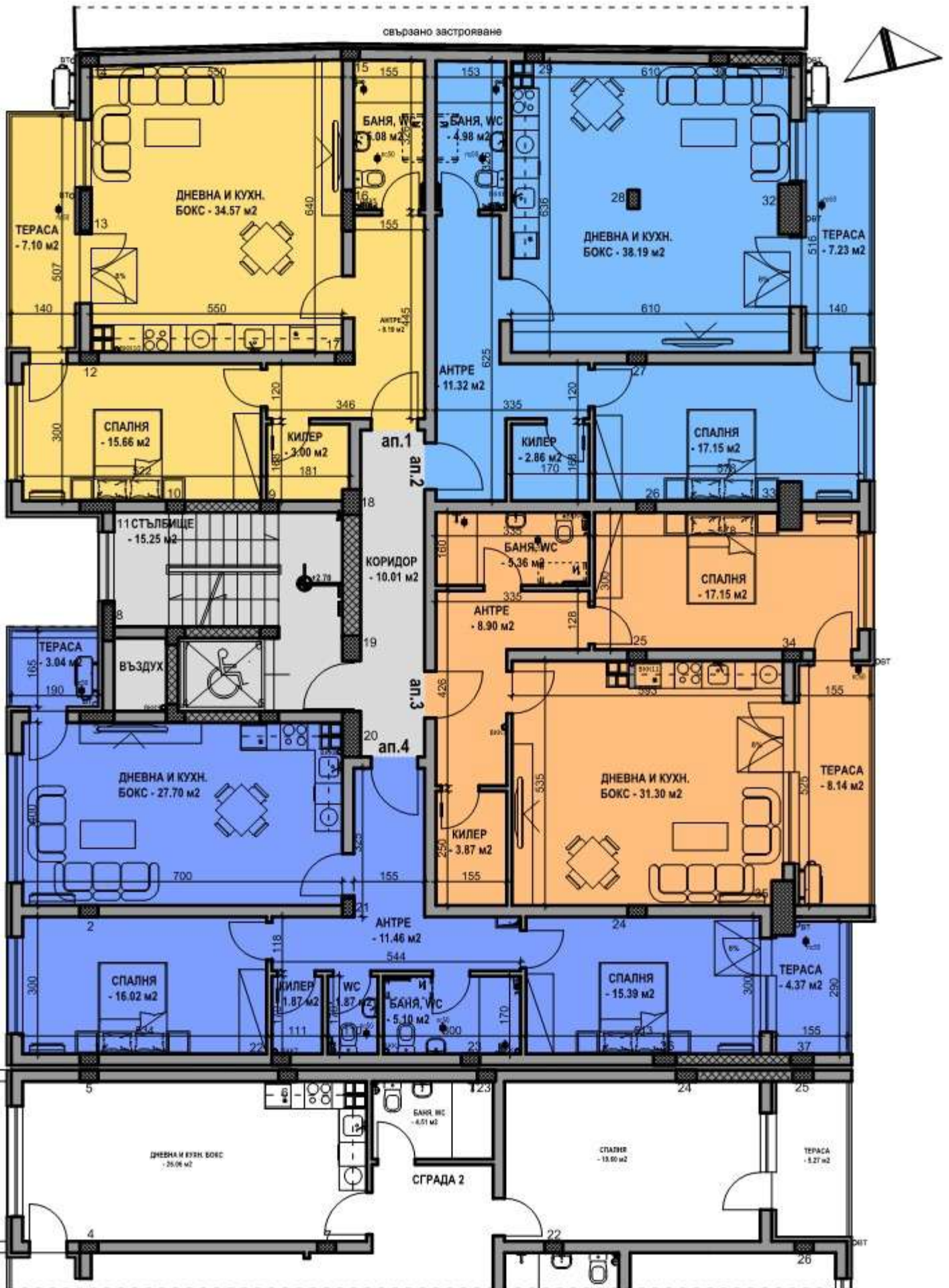
СГРАДА 1: РАЗПРЕДЕЛЕНИЕ ВТОРИ ЕТАЖ - КОТА +2.70
