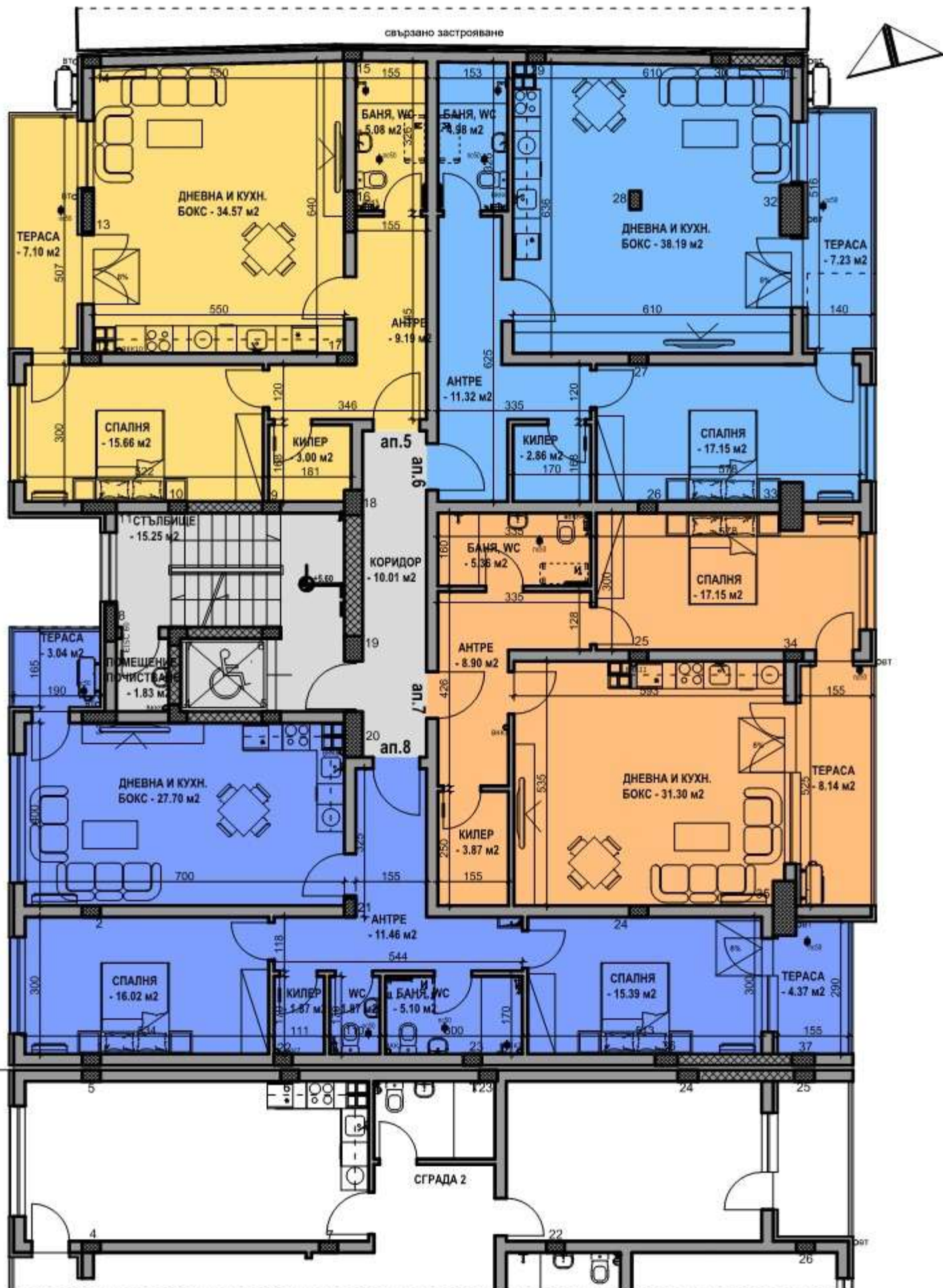
СГРАДА 1: РАЗПРЕДЕЛЕНИЕ ТРЕТИ ЕТАЖ - КОТА +5.60
