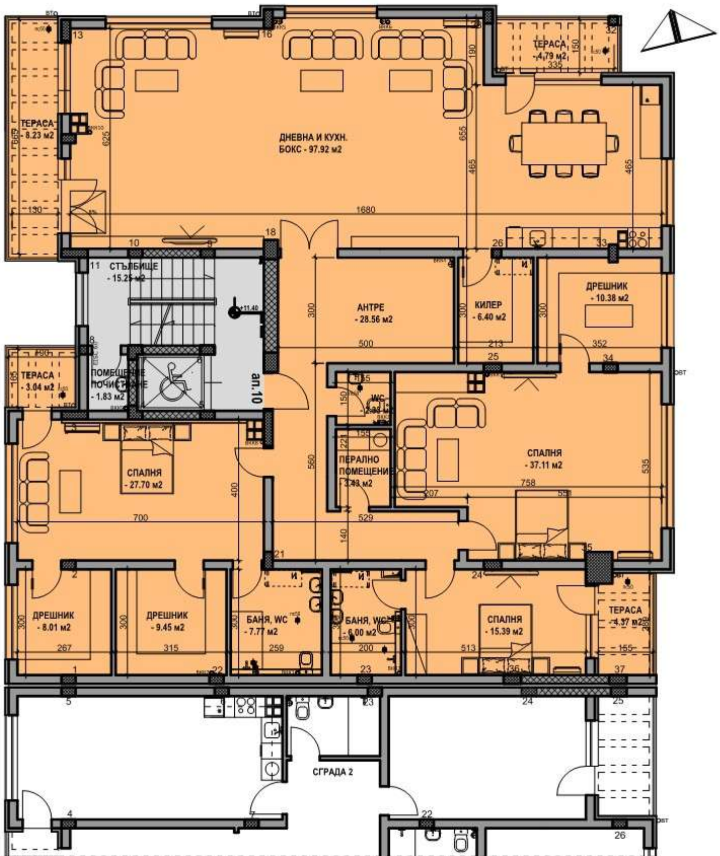
СГРАДА 1: РАЗПРЕДЕЛЕНИЕ ПЕТИ ЕТАЖ - КОТА +11.40
