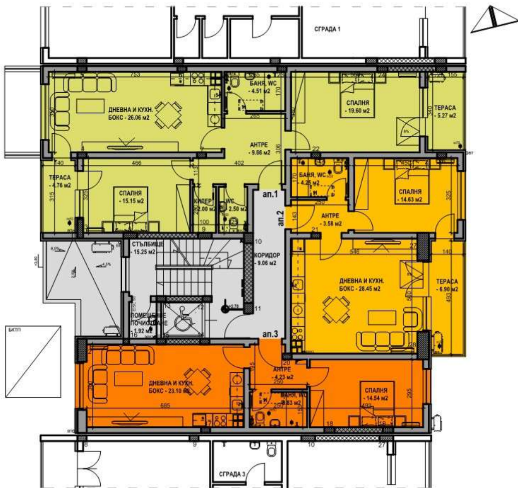
СГРАДА 2: РАЗПРЕДЕЛЕНИЕ ВТОРИ ЕТАЖ - КОТА +2.70
