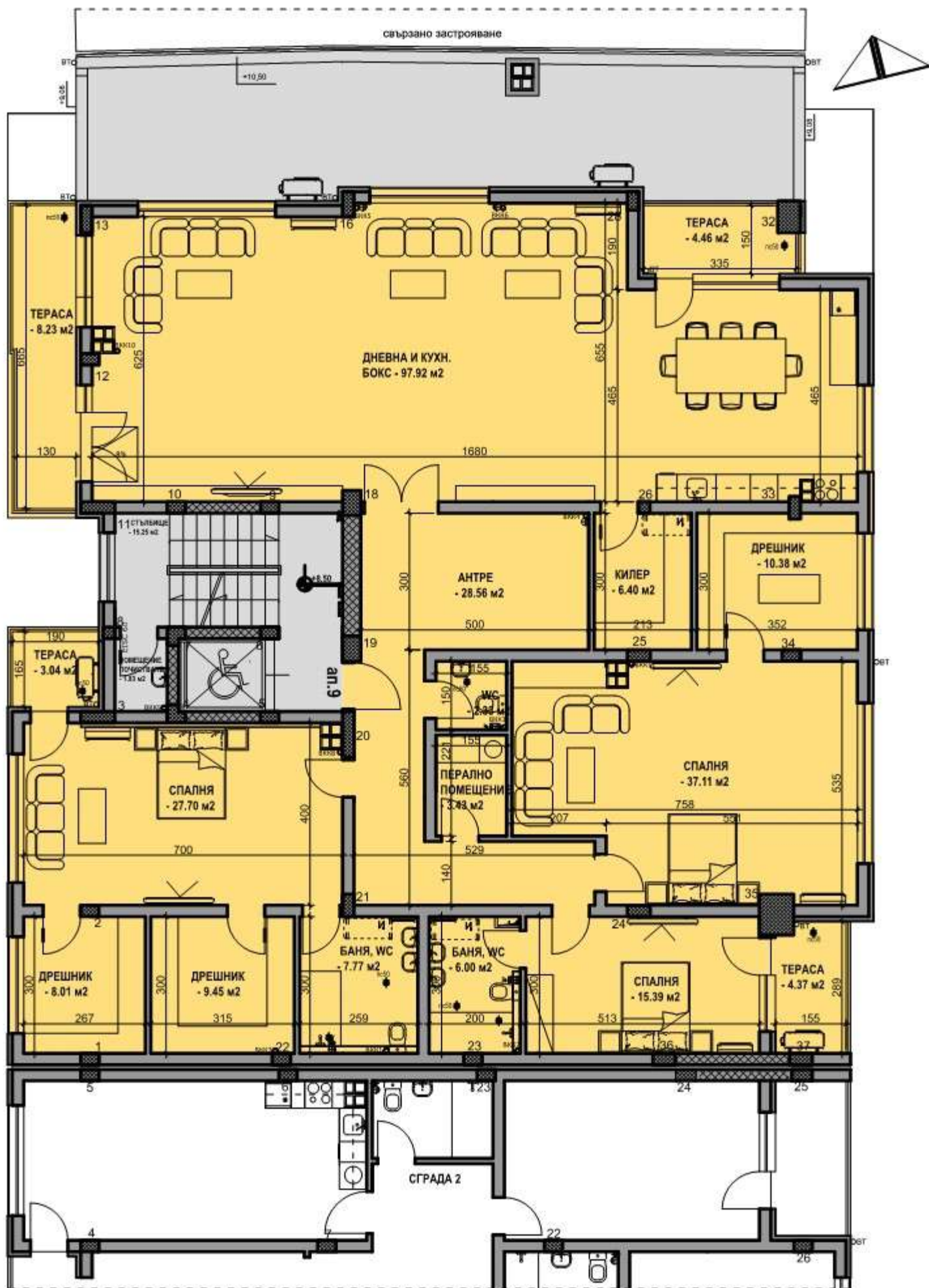
СГРАДА 1: РАЗПРЕДЕЛЕНИЕ ЧЕТВЪРТИ ЕТАЖ - КОТА +8,50
